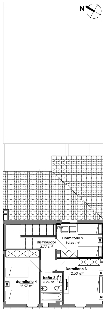
Planta Primera
